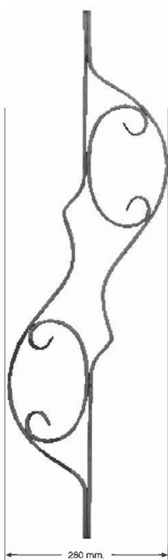
4-5414 L: 950 mm. Ø 14 mm. (dos pletinas de 14x7).
