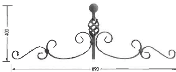
4-2302 Medidas: 890 x 400 mm. M: 12 x 6 mm.
